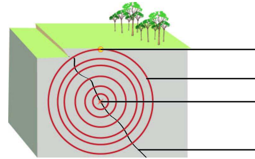
Schéma représentant l'origine d'un séisme et sa propagation
