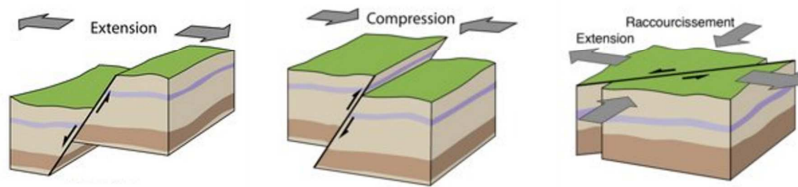
Schéma représentant l'origine d'un séisme et sa propagation
