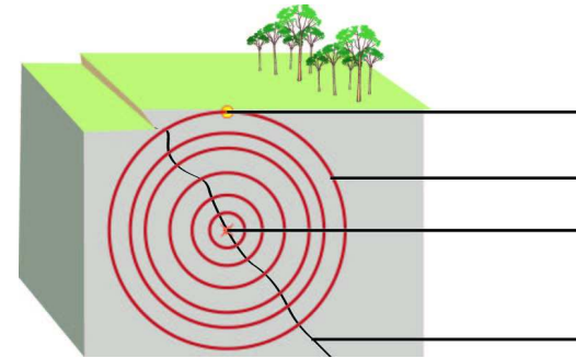
Schéma représentant l'origine d'un séisme et sa propagation
