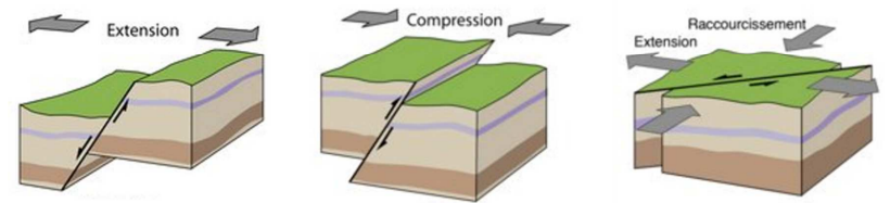
Schéma représentant l'origine d'un séisme et sa propagation
